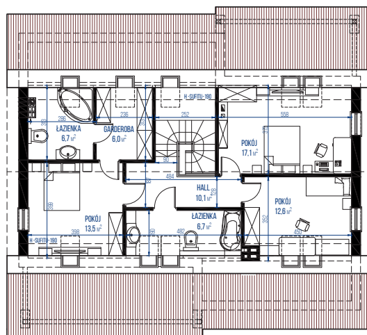
RZUT PODDASZA: 87,0m 2
