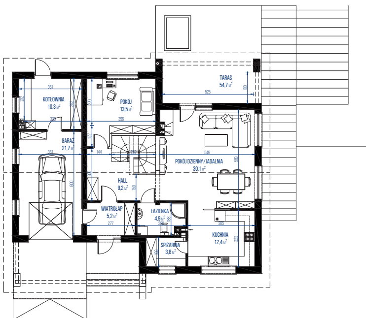
RZUT PARTERU: 111,1m 2
