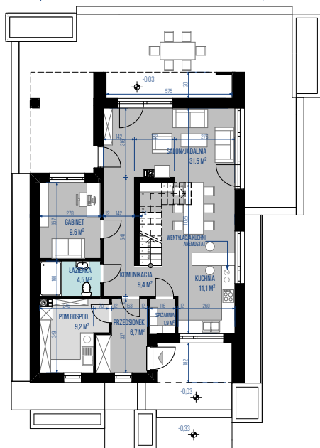
RZUT PARTERU: 83,6m 2
