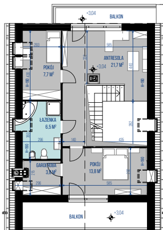
RZUT PODDASZA: 72,9m 2
